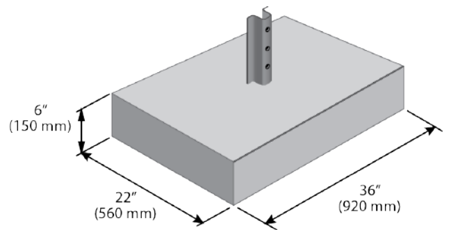
BASE DE BÉTON RECTANGULAIRE : B-250
