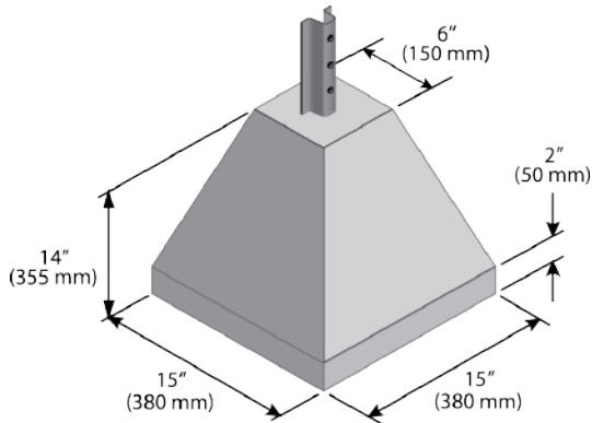
BASE DE BÉTON PYRAMIDALE : B-115
