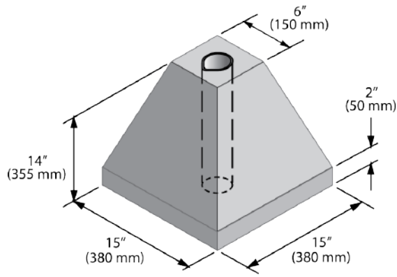
BASE DE BÉTON PYRAMIDALE
