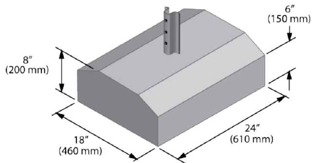
BASE DE BÉTON RECTANGULAIRE
