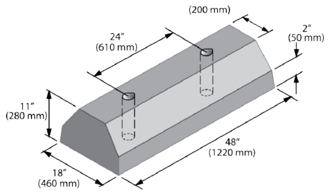
BASE DE BÉTON RECTANGULAIRE
