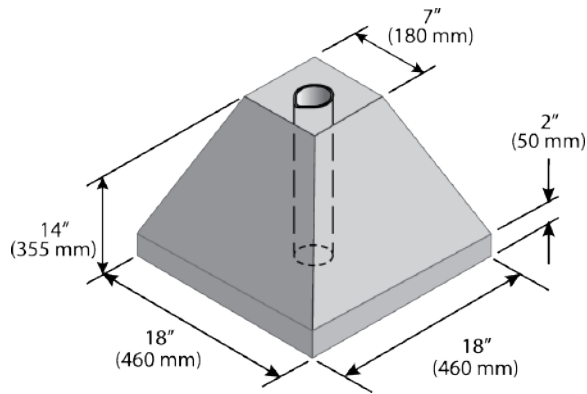
BASE DE BÉTON PYRAMIDALE
